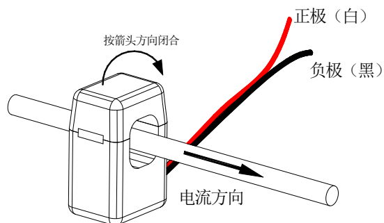
开合式互感器安装方式
